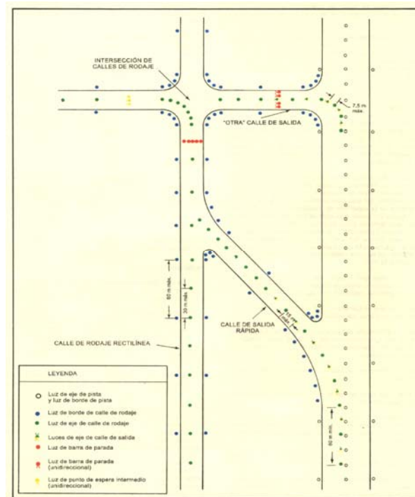
Figura 5-24. Luces indicadoras de calle de salida rápida
